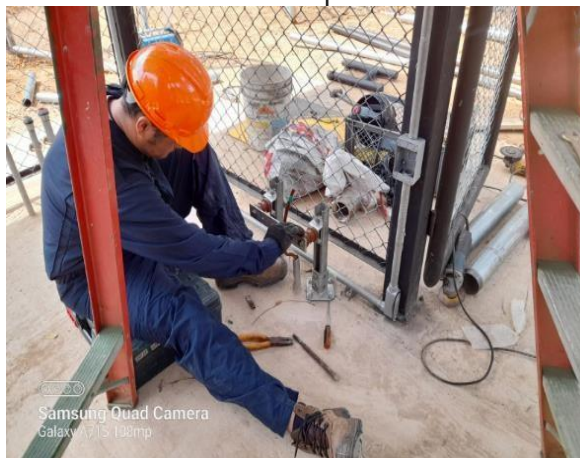
Instalación de tubería IMC, barraje equipotencial y accesorios eléctricos Casetas Bombas 1 y 2 CPF Cup.
