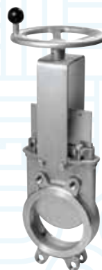
| Modelo EK Unidireccional tipo wafer
