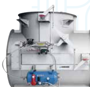
| Modelo DI Dámper distribuidor en forma de T (3 vías) de sección redonda o cuadrada
