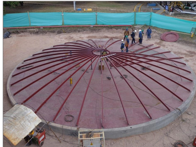
Montaje de la estructura del techo
