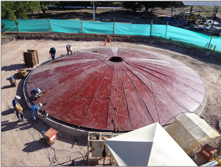
Montaje láminas de techo
