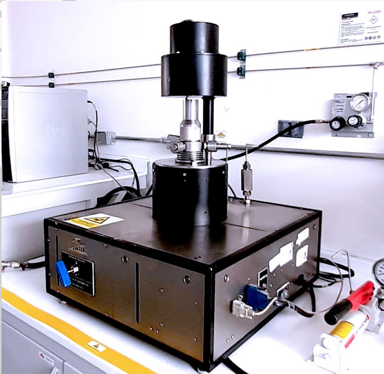
Viscosímetro HTHP - OFITE 77
